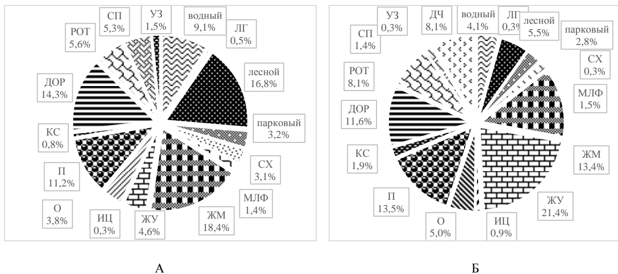
Рис.1. Соотношение различных типов климатопопов на территории г.Минска (А) и Витебска (Б). Условные обозначения типов климатопопов: в незастроенной части города: ЛГ – лугопарковые, СХ – сельскохозяйственные, МЛФ – малые ландшафтные формы (скверы, бульвары и др.), РОТ – резервные озелененные территории; в застроенной части: ЖМ– жилая многоэтажная, ЖУ – жилая усадебная, ДЧ – дачная, О – общественная, П – производственная, КС – коммунально-складская застройки, ИЦ – исторический центр, СП – спецтерритории, ДОР – дорожная инфраструктура, УЗ – участки незавершенного строительства.
