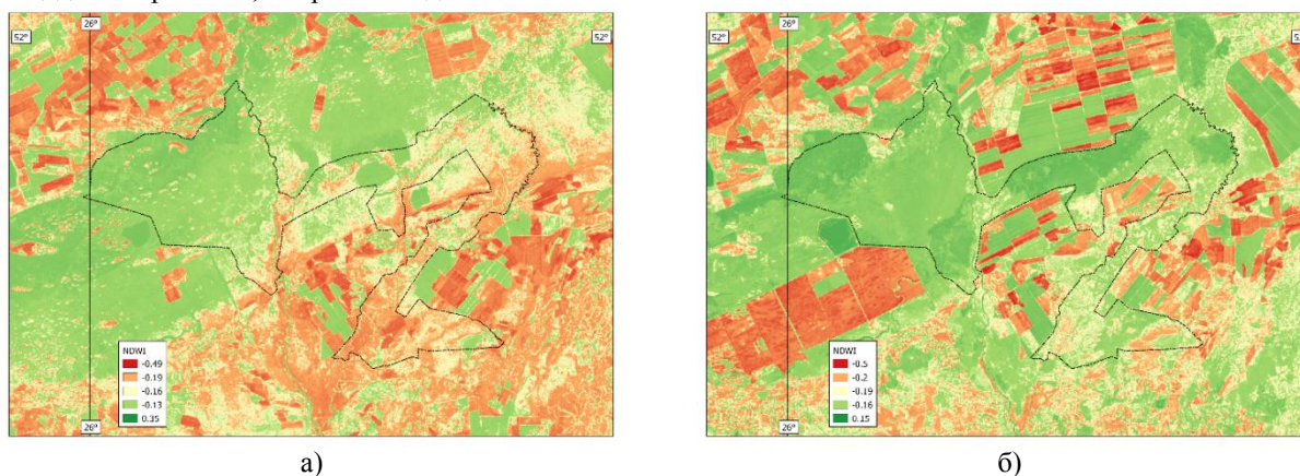
Рис. 2 – Индекс NDWI на апрель а) 1986 г., б) 2020 г.
