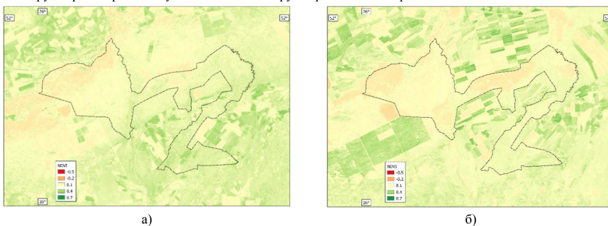
Рис. 1 – Индекс NDVI на апрель а) 1986 г., б) 2020 г.
