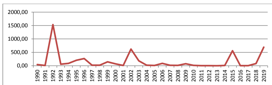
Рис. 2 – Выбросы ПГ от лесных пожаров, тыс. т CO 2 -эquiv.
