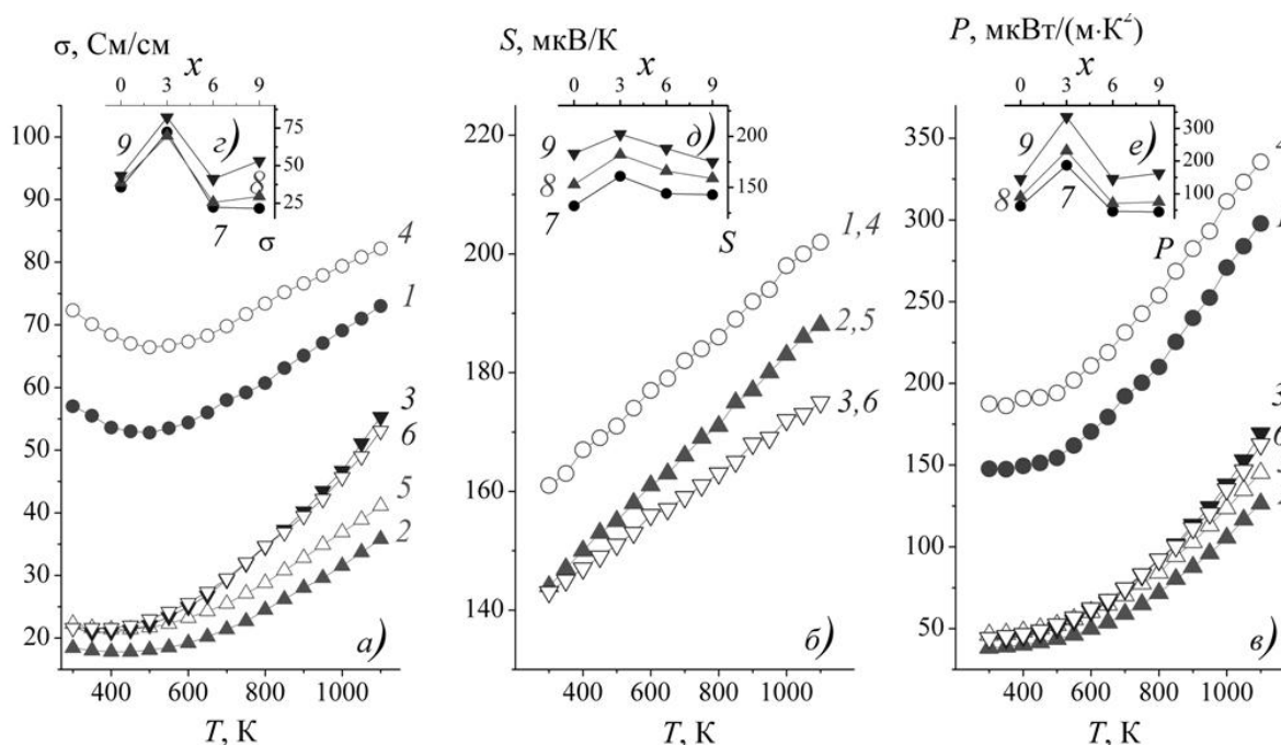
Рис. – Температурные (а–в) и концентрационные (z–e) зависимости удельной электропроводности ( \sigma ) (а, z), коэффициента термо-ЭДС ( S ) (б, d) и фактора мощности ( P ) (в, e) керамики состава \text{Ca}_3\text{Co}_4\text{O}_{9+\delta} + x мас.% Cu, спеченной при 1273 К: x = 3 (1, 4), 6 (2, 5) и 9 (3, 6) в направлении параллельно (1–3) и перпендикулярно (4–6) оси прессования при температурах 300 К (7), 700 К (8) и 1100 К (9)
