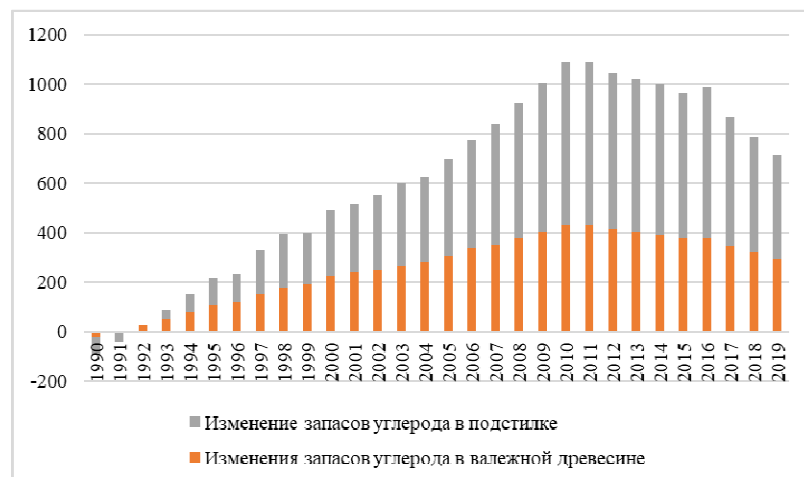
Рисунок 1. – Изменение запасов углерода в мертвой биомассе, тыс. т С
